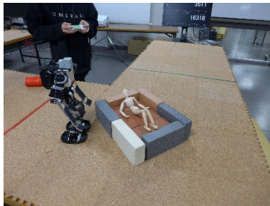
(4) 要救助者人形は規定された姿勢でベッドの上に設置、ベッドを囲むようにガレキが配置されている。
